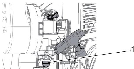
1. Gaasiasendi hoob
