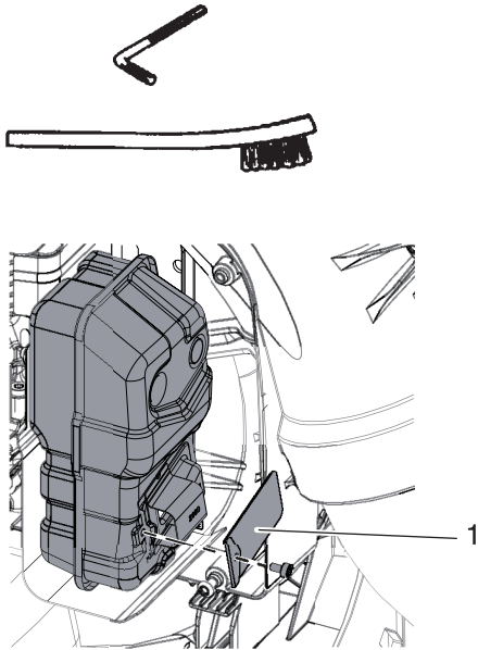
1. Sädemepüüdja ekraan
