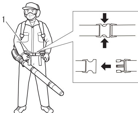
1. Puusavöö
