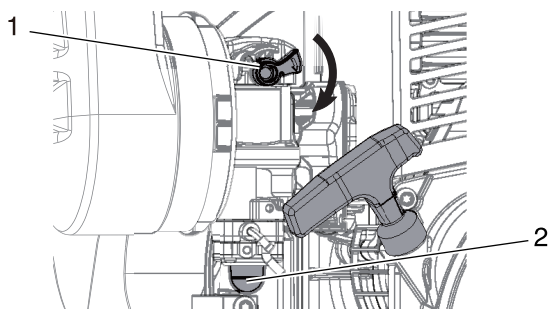
1. Õhuklapi hoob
