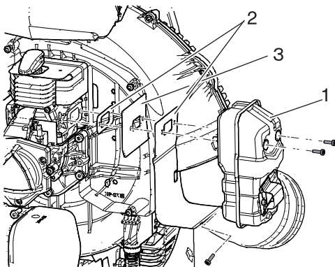
1. Summuti
