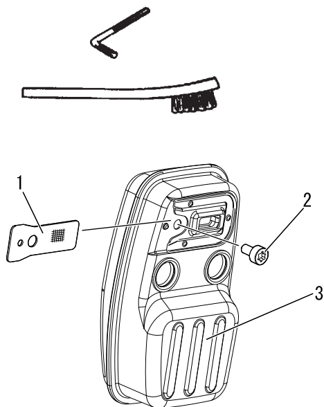
1. Sädemepüüdja ekraan
