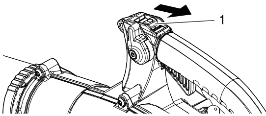
1. Stopplüliti
