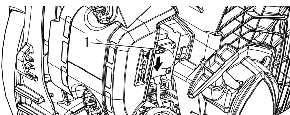
1. Õhuklapp
