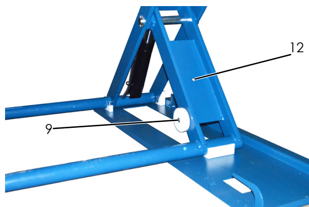
9 Assale 12 Conservazione dell'assale 019
