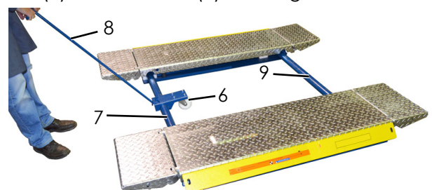
6 Lenkrolle
