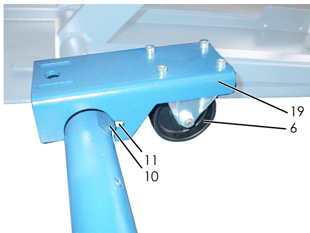
6 Rullo di rinvio 10 Trascinatore 11 Asola 19 Supporto rullo di rinvio 005
