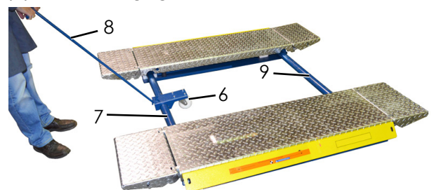
6 Guide roller
